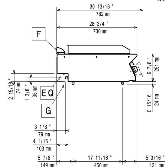
Boční
